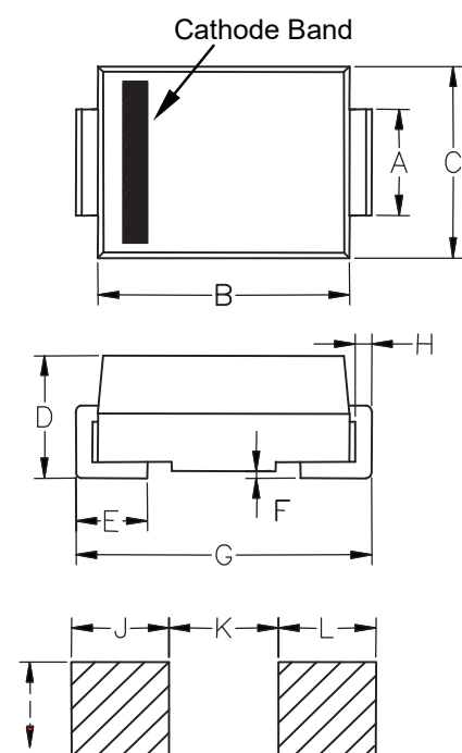
DO-214AB (SMC)
