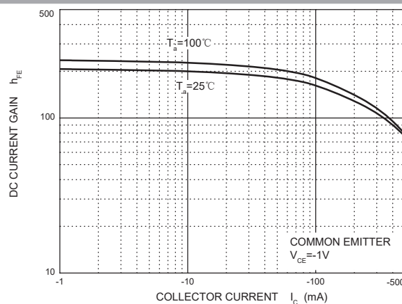
Fig. 2 h_{FE} - I_c
