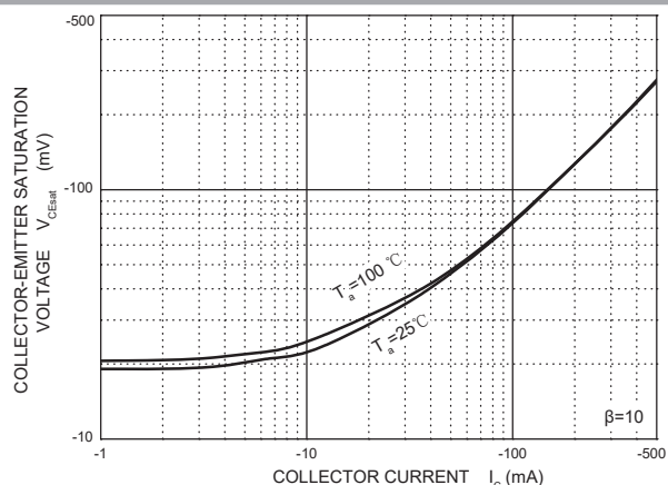
Fig. 3 V_{CE(sat)} - I_c
