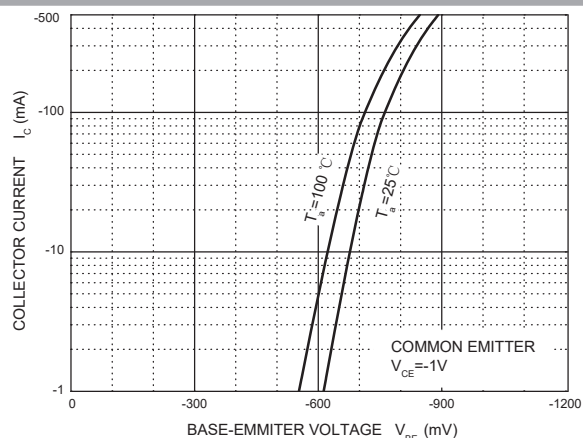
Fig. 5 I_c - V_{BE}
