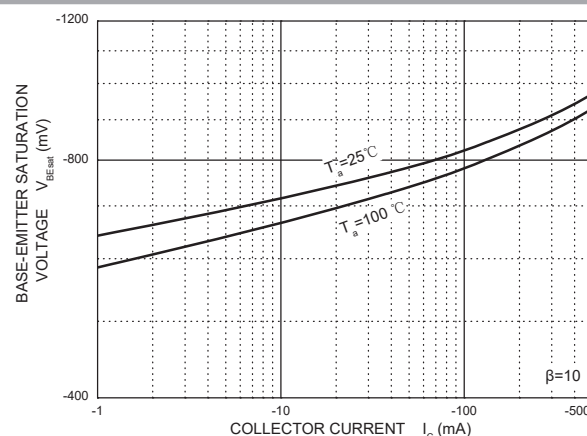
Fig. 4 V_{BE(sat)} - I_c
