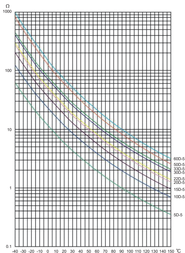
电阻-温度曲线 Resistance-Temperature Curve
